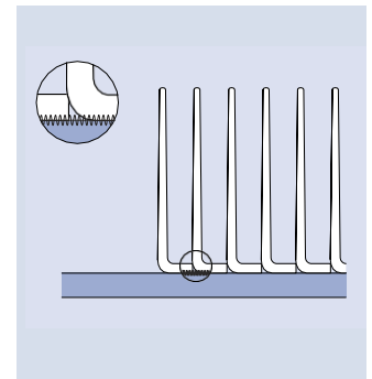
KL Fin (Knurled L Fin)
